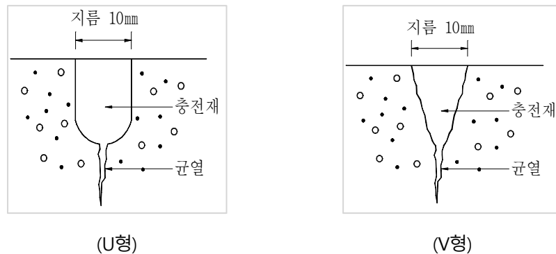
[그림 7.3.4] 철근이 부식되지 않은 경우의 충전공법
